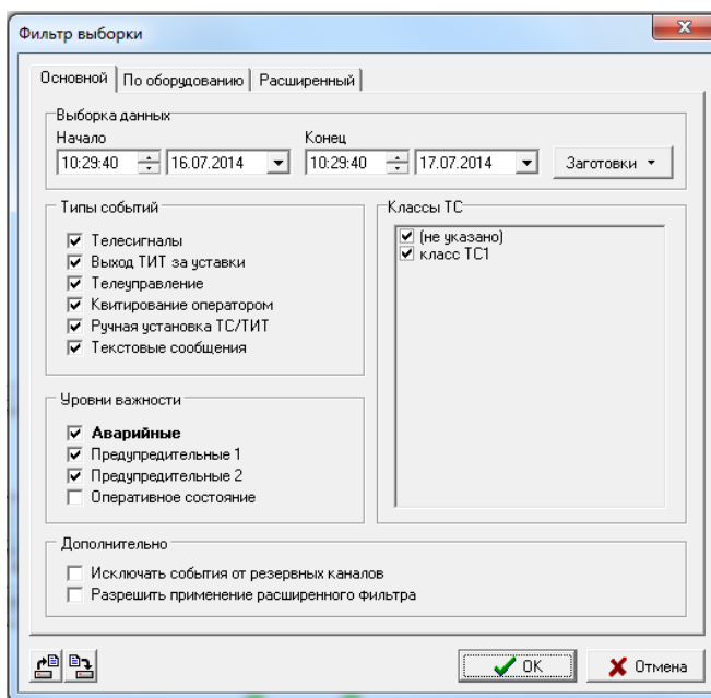
Рис. 7.8 Окно настройки фильтра выборки ретроспективы событий
