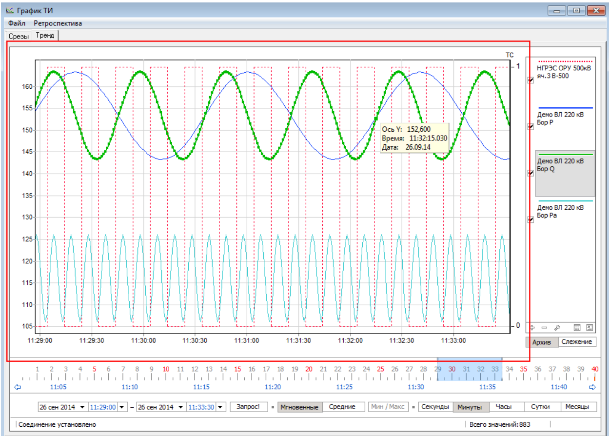
Рис. 6.2 Просмотр графиков из SQL БД (закладка «Тренд», область отображения графика)
