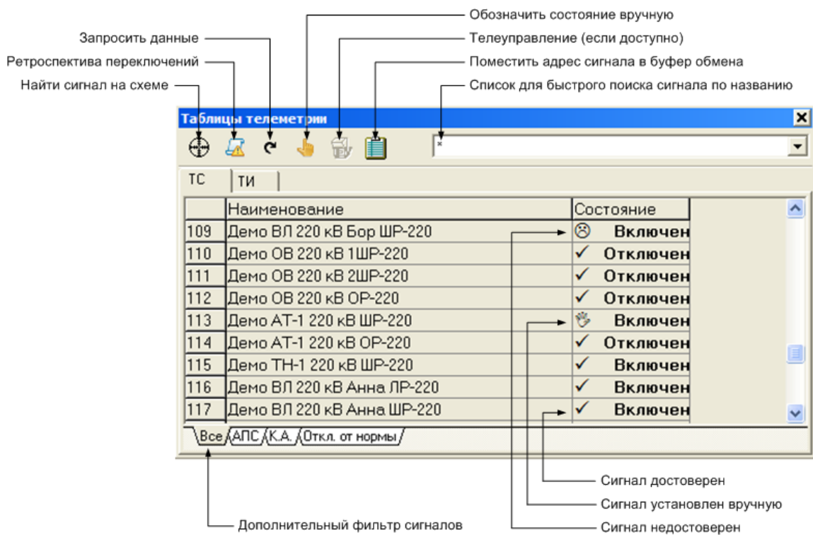
Рис. 5.5 Окно просмотра таблицы сигналов
