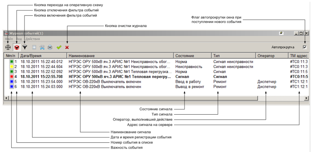
Рис. 4.4 Окно просмотра журнала событий
