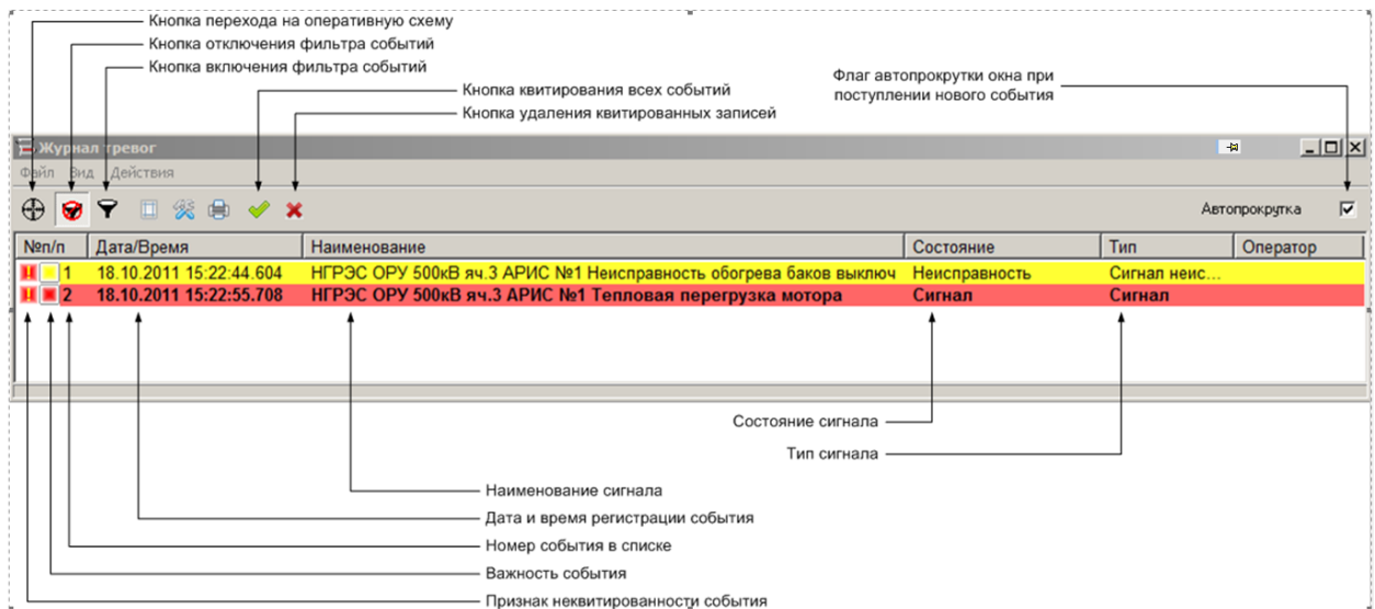
Рис. 4.5 Окно просмотра журнала тревог
