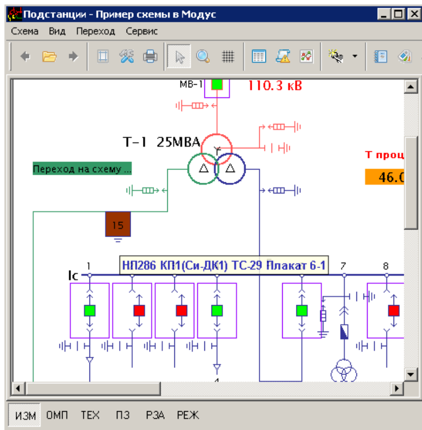
Рис. 7.25 Оперативная схема с установленным переносным заземлением
